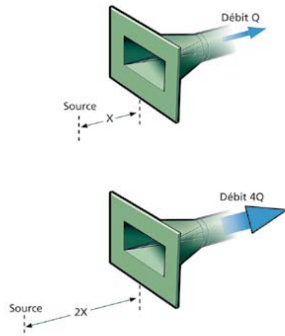
Figure 11 : Influence de la distance du capteur sur le débit d'aspiration
