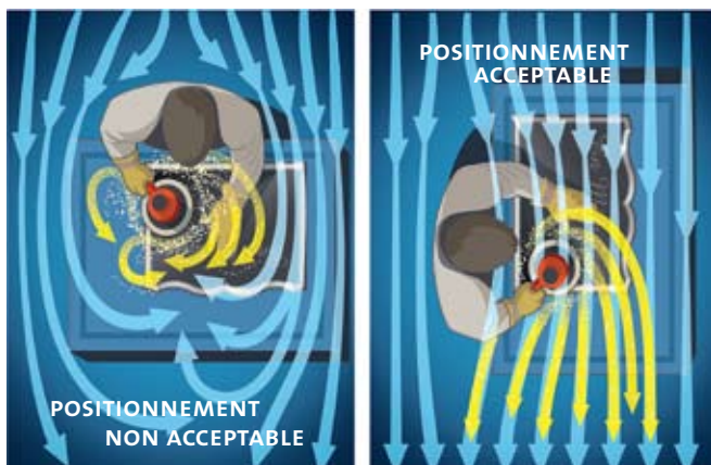
Figure 6 : Importance du positionnement adéquat du travailleur
