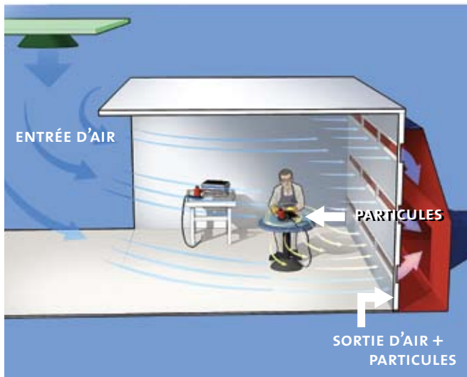
Figure 5 : Enceinte à flux d'air horizontal
