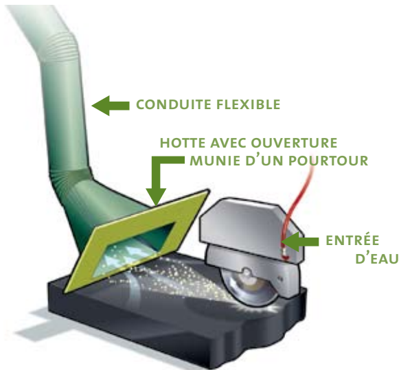
Figure 10 : Outil muni d'une conduite flexible
