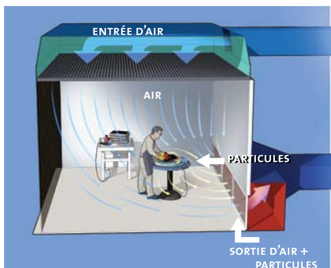
Figure 4 : Enceinte à flux d'air oblique
