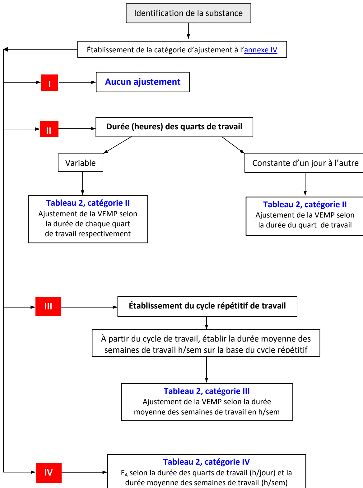
Figure 1 : Démarche d'ajustement d'une VEMP
