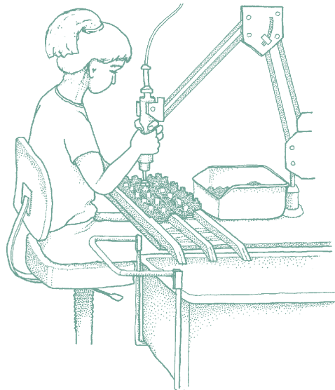
Fig. 4.8 Vue du poste réaménagé. Notez le rapprochement des rails et l'installation d'un pantographe qui diminuent les contraintes au niveau de l'épaule et les exigences de force lors du vissage.
