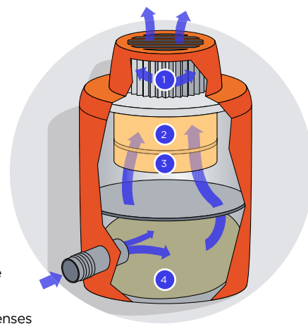
FIGURE 2 Aspiration avec filtre HEPA
