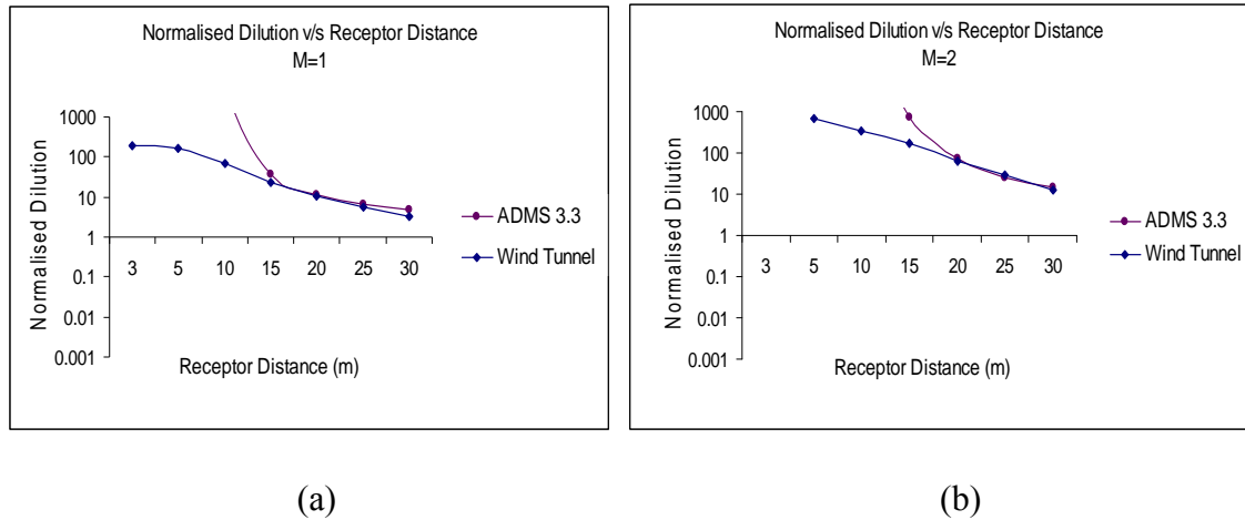
Figure 5.21 Dilution normalisée par rapport à la distance des récepteurs pour une cheminée haute de 7 m par vent à 45 degrés azimut
