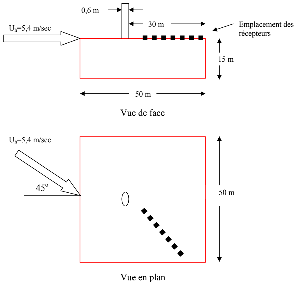
Figure 5.17 Vent à angle de 45^\circ sur un bâtiment de faible hauteur
