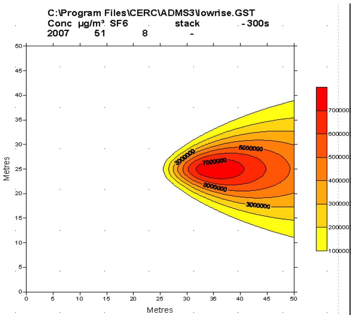
Figure A 4 Grille montrant le tracé de contours pour un bâtiment de faible hauteur surmonté d'une cheminée haute de 3 mètres
