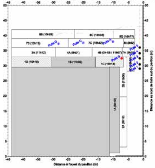
Teneur en CO dans le sol 100 @ 130 min. après les sautages 1C & 1D
