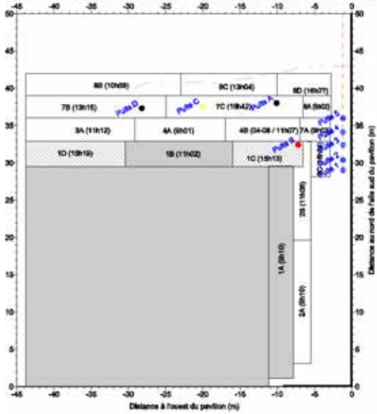
Teneur en CO dans le sol 70 @ 100 min. après les sautages 1C & 1D
