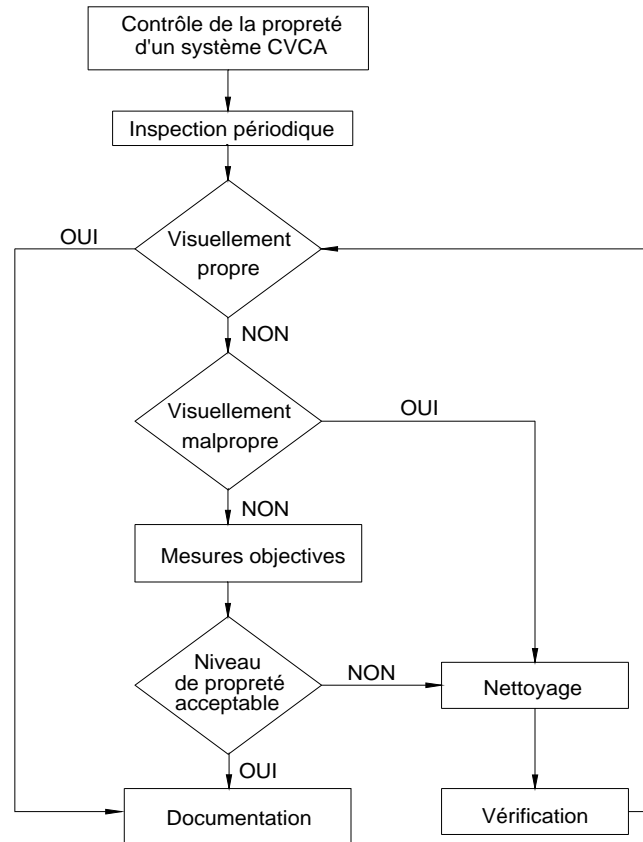
Figure 7 : Diagramme résumant les procédures à suivre pour la maintenance d'un système CVCA
