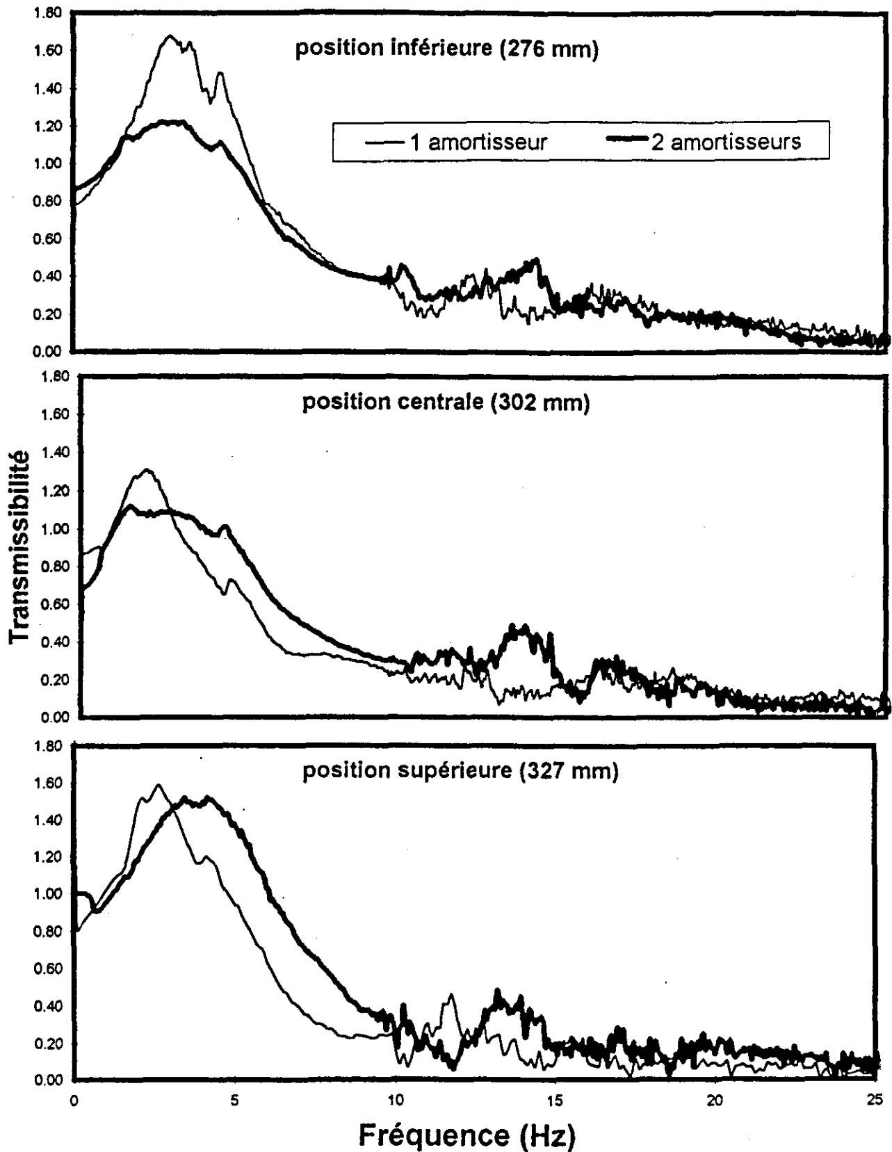
Figure 18: Influence de l'amortissement du siège Recaro CL-1 pour un réglage permettant la moitié de la course (réglage #2) et différentes positions en hauteur.
