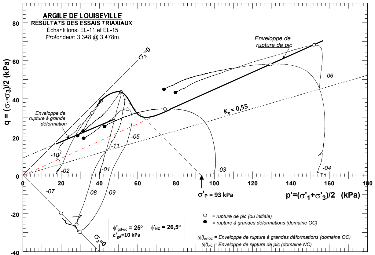
Figure 44. Argile de Louiseville : Résultats des essais triaxiaux - cheminement de contraintes et enveloppes de rupture. Domaine OC = domaine surconsolidé; Domaine NC = domaine normalement consolidé
