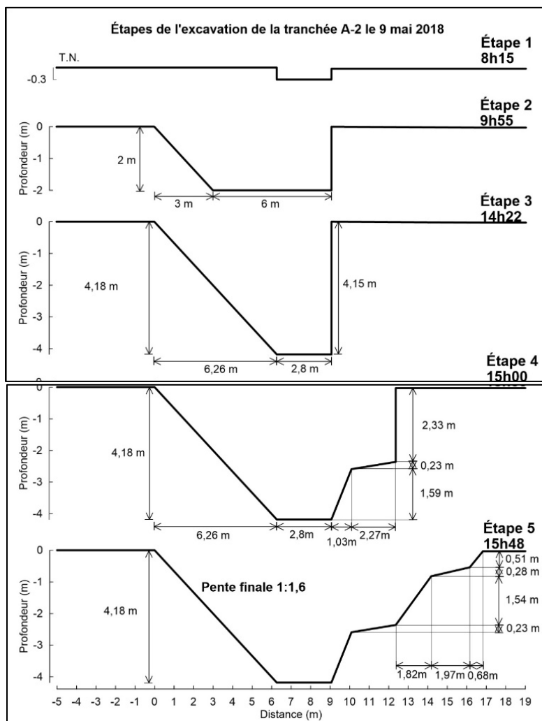
Figure 28. Étapes chronologiques de l'excavation de la tranchée A-2 : vues en coupe. De Étude expérimentale de deux excavations à Louiseville , par S. Dourlet, 2020. ©S. Dourlet, 2020. Reproduit avec permission.
