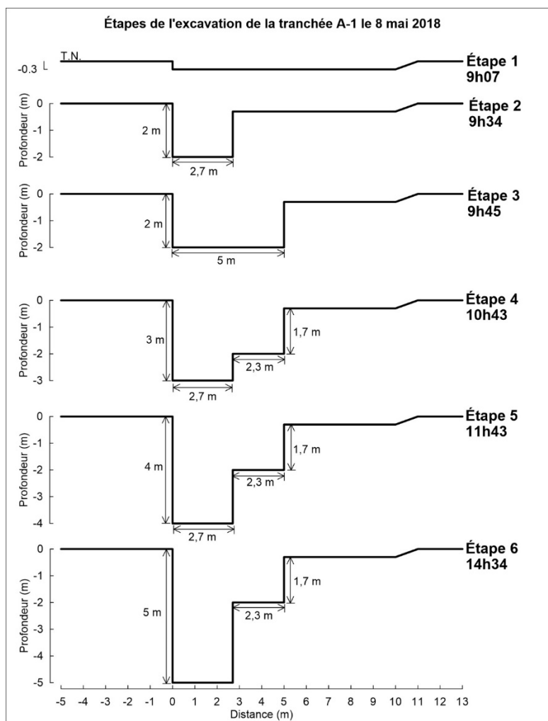
Figure 25. Étapes chronologiques de l'excavation de la tranchée A-1 : vue en coupe. De Étude expérimentale de deux excavations à Louiseville , par S. Dourlet, 2020. ©S. Dourlet, 2020. Reproduit avec permission.
