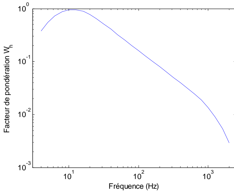
Figure 6. Facteur de pondération W_h en fonction de la fréquence
