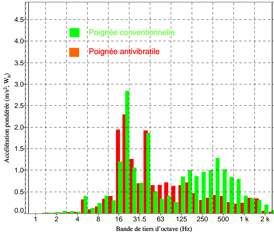
Figure 24. Exemple d'atténuation d'une poignée antivibratile, axe y
