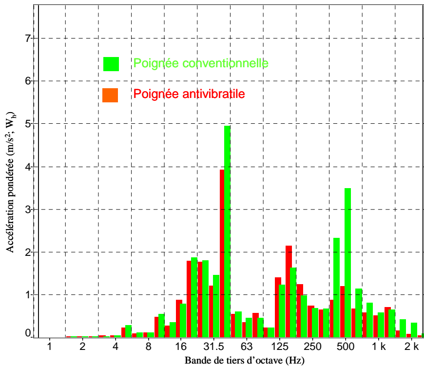
Figure 23. Exemple d'atténuation d'une poignée antivibratile, axe x
