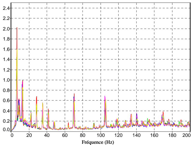
Figure 13. Répétabilité de 5 essais, axe y
