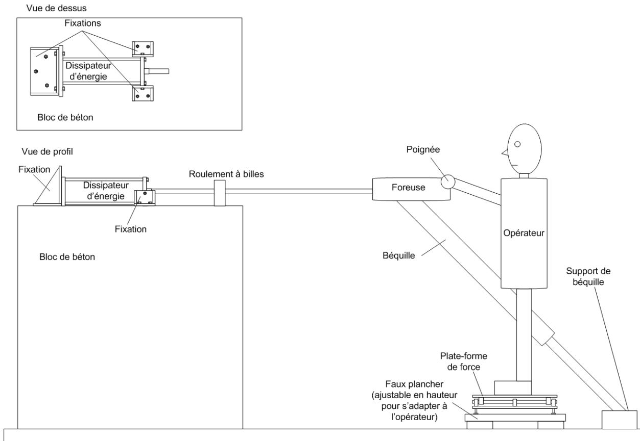
Figure 3. Schéma global du banc d'essai
