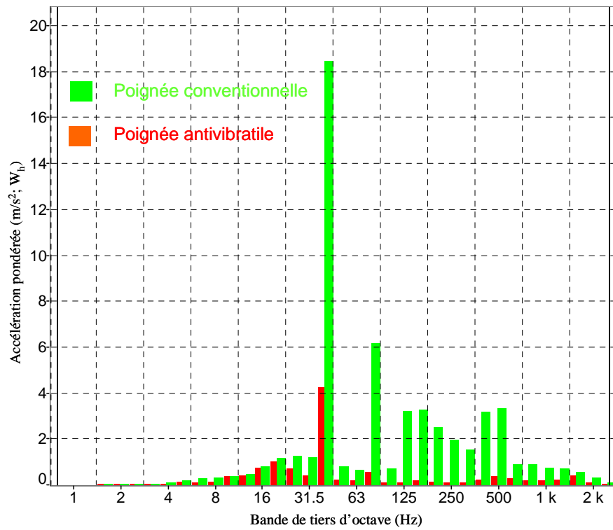
Figure 25. Exemple d'atténuation d'une poignée antivibratile, axe z
