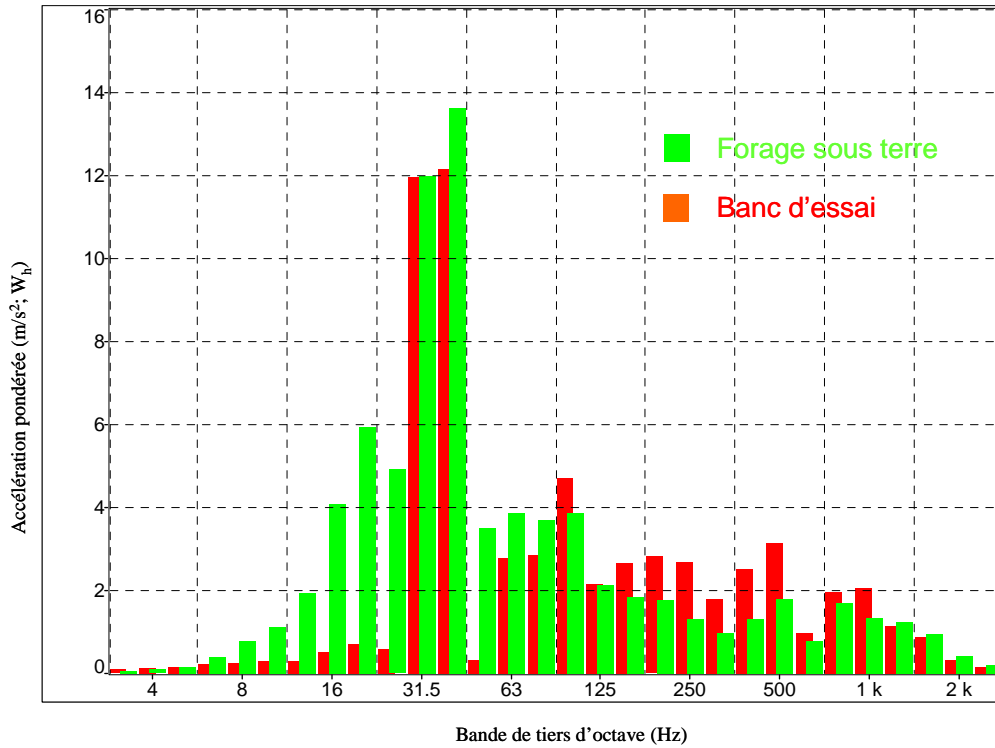
Figure 21. Validation du banc d'essai, axe z
