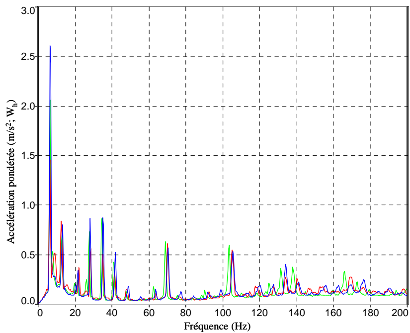
Figure 16. Répétabilité de 3 séries de mesure, axe y
